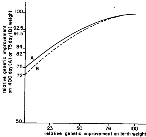
FIG. 1. — Some results about selection indices with restriction on birth weight applied to bulls of terminal crossing Résultats concernant l'application aux taureaux de croisement terminal d'indices de sélection avec contrainte sur le poids à la naissance
